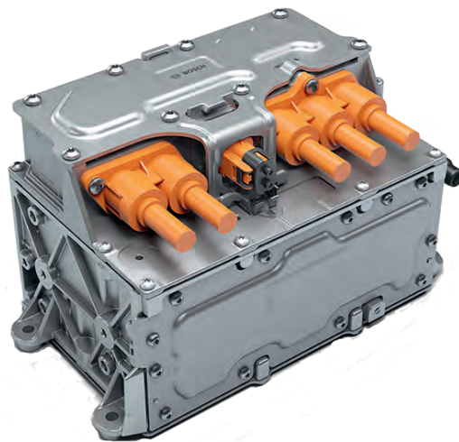
Abb.16: Exemplarische Darstellung einer im Projekt betrachteten Leistungselektronik (Quelle: Bosch)
